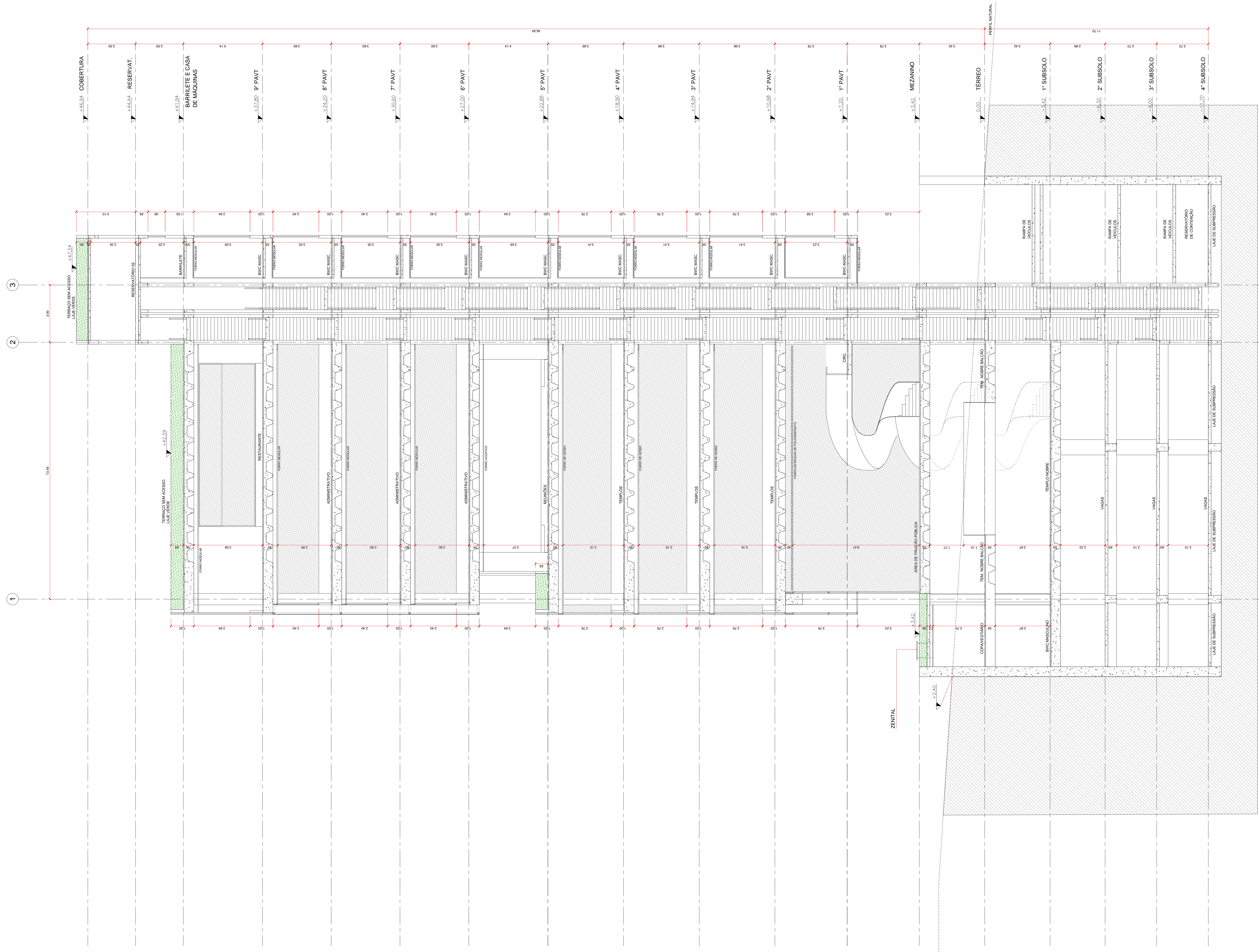
RF: 0,00 = 97,00 (TOPOGRÁFICO) CORTE AA ESCALA 1/75
