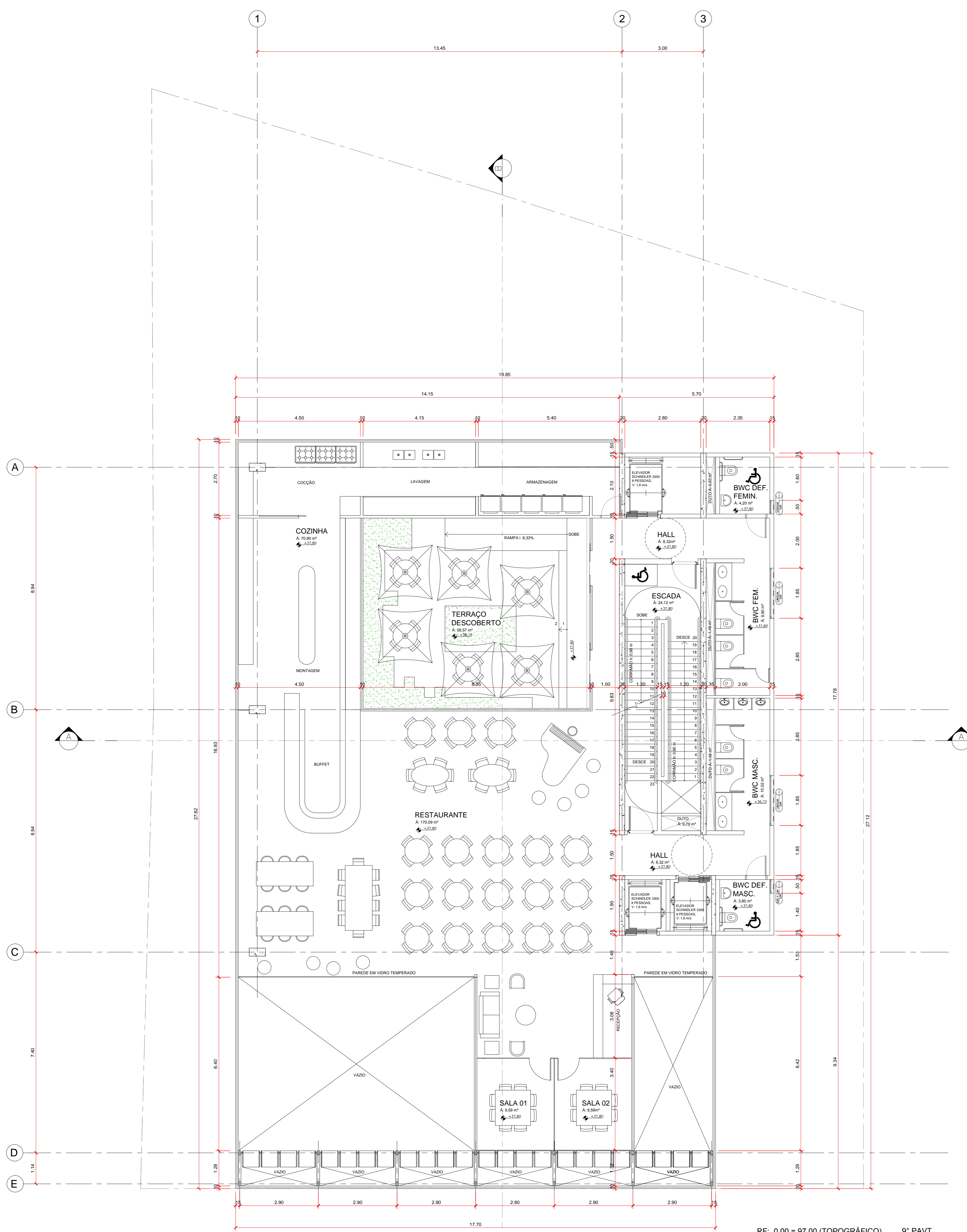
RF: 0,00 = 97,00 (TOPOGRÁFICO) 9º PAVT ESCALA 1:50 OBS: AS ÁREAS EM PLANTA SÃO ÁREAS ÚTIS, SEM PAREDES
