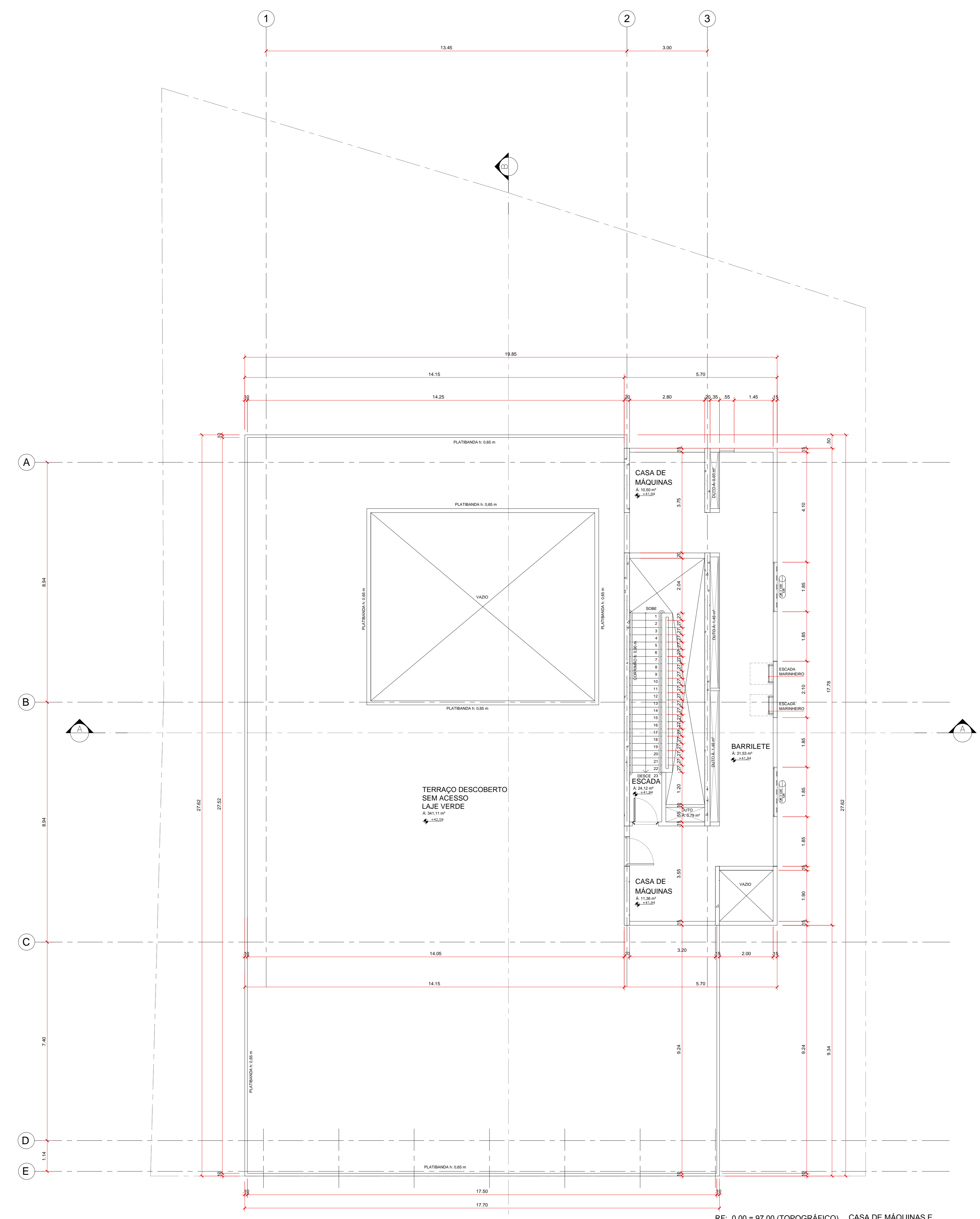
RF: 0,00 = 97,00 (TOPOGRÁFICO) CASA DE MÁQUINAS E BARRILETE ESCALA 1:50 OBS: AS ÁREAS EM PLANTA SÃO ÁREAS ÚTIS, SEM PAREDES
