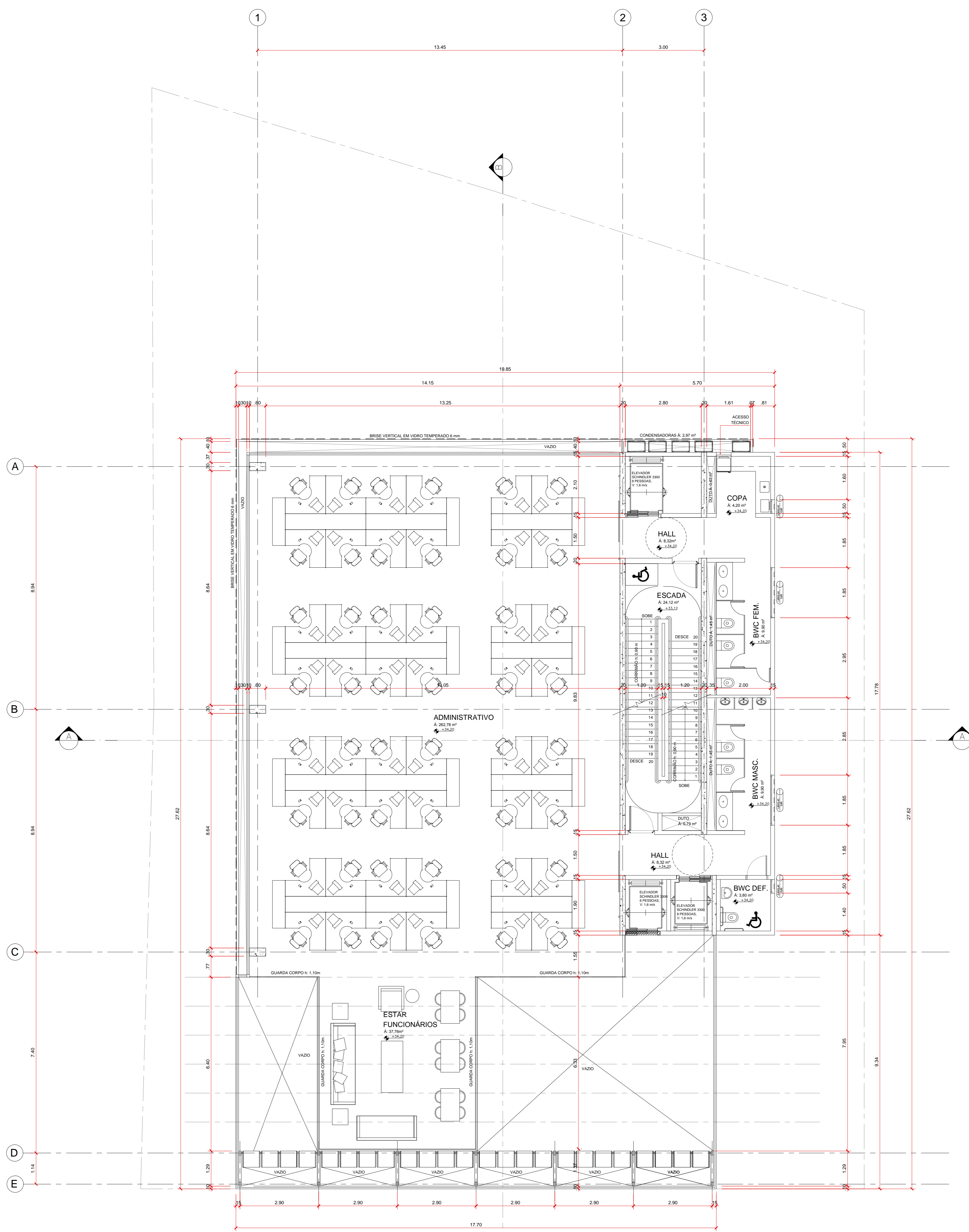
RF: 0,00 = 97,00 (TOPOGRÁFICO) 8º PAVT ESCALA 1:100 OBS: AS ÁREAS EM PLANTA SÃO ÁREAS ÚTEIS SEM PAREDES
