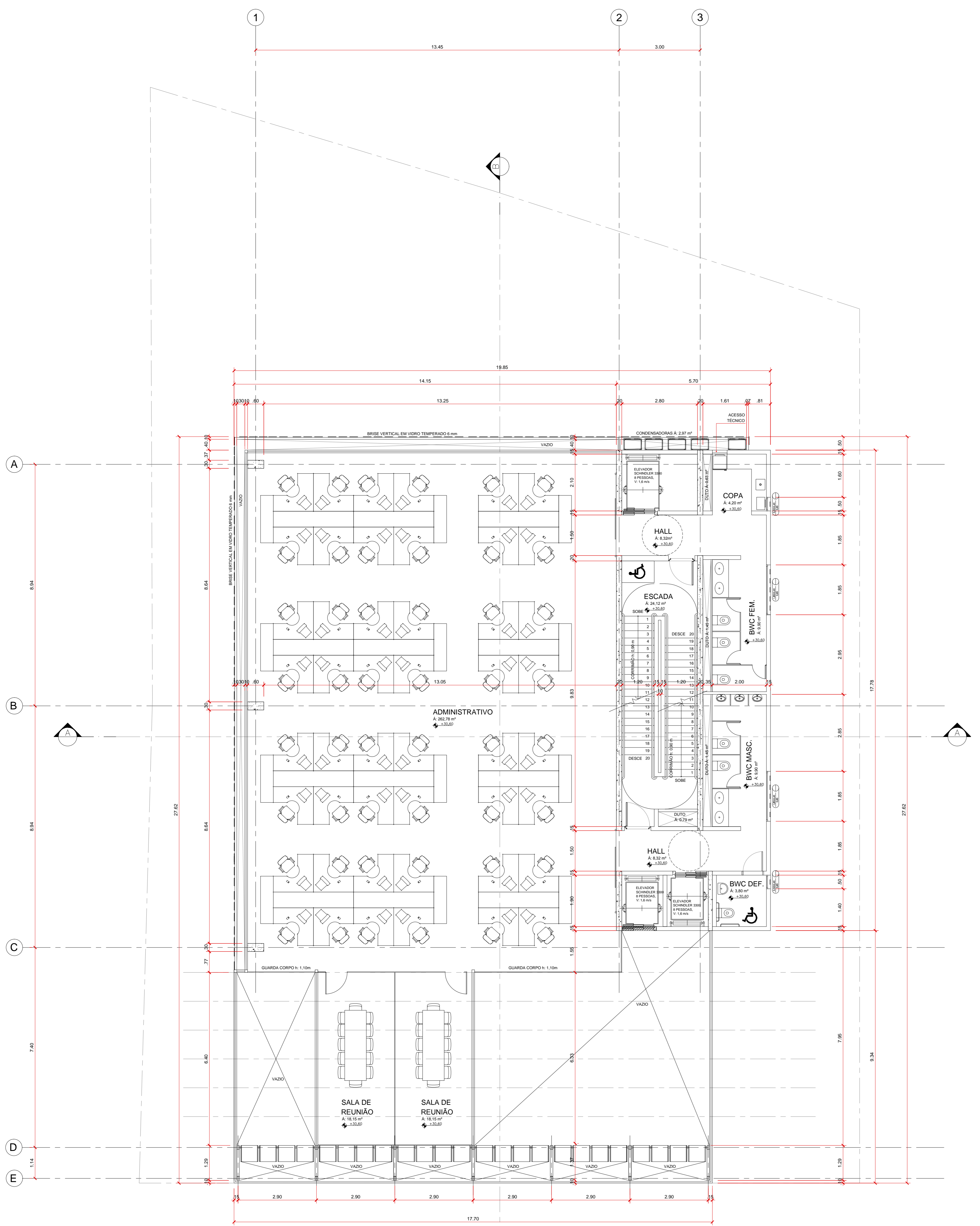
RF: 0,00 = 97,00 (TOPOGRÁFICO) 7º PAVT ESCALA 1:100 OBS: AS ÁREAS EM PLANTA SÃO ÁREAS ÚTEIS SEM PAREDES
